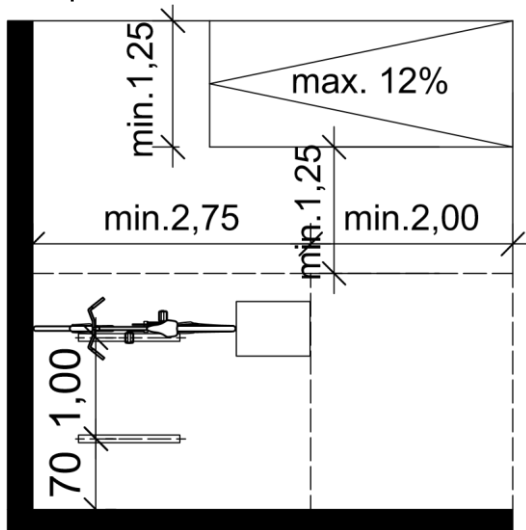
Beispiel Fahrradständer mit Mindestmaßen für Sonderräder
