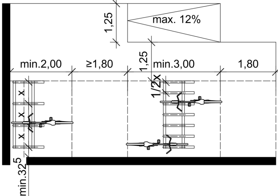
Beispiel Fahrradständer mit Mindestmaßen
